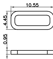
防水圈图示
